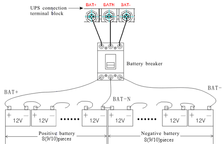
UPS 10-30 kVA
