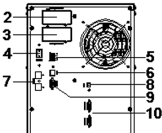
Interfacce di comunicazione (30-40 kVA, vista posteriore)
