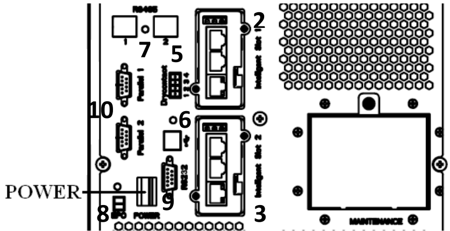
Interfacce di comunicazione (10-20 kVA, vista posteriore)
